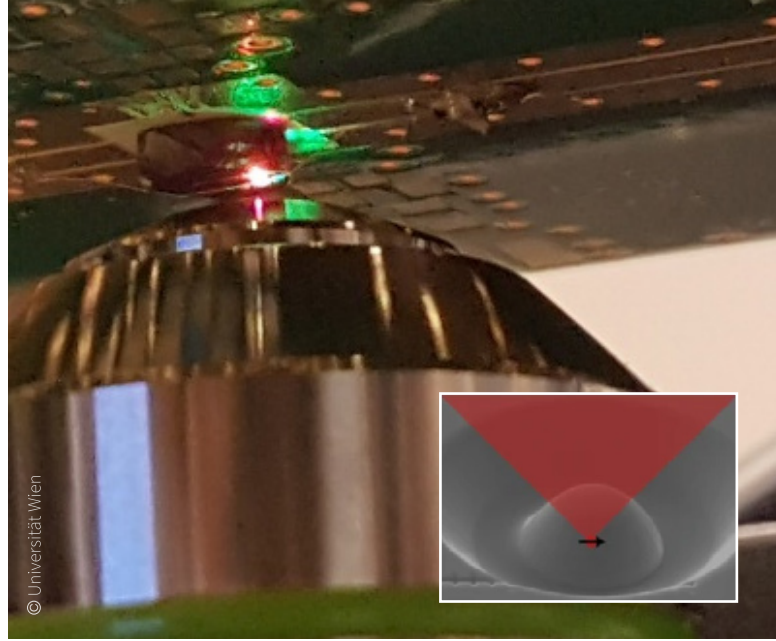
Abb. 3: Zur Steigerung der Photonenabgabe werden Mikrolinsen (0,01 mm) direkt über dem Farbzentrum im Diamanten erzeugt. Für Quantensensorik werden dotierte Diamanten mit mikroelektronischen Komponenten integriert.
